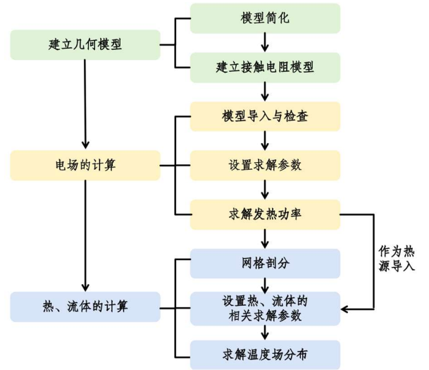
图2 GIS 三工位开关热分析仿真计算流程图
