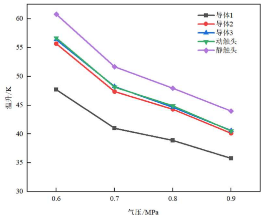
(b) 0.6~0.9 MPa 下导体和动静触头随气压增大的温升情况
