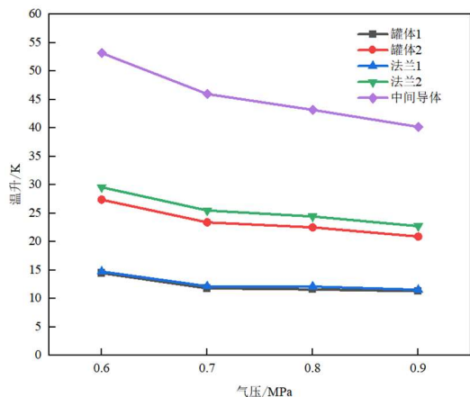
(a) 0.6~0.9MPa 下罐体、法兰和中间导体随气压增大的温升情况
