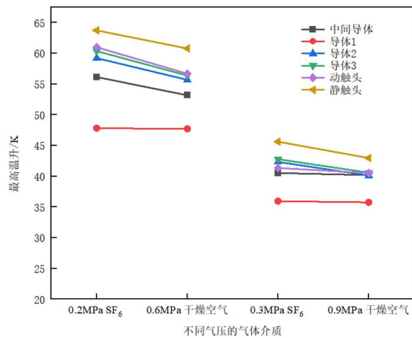
图 11 不同气压的气体介质下关键部件的最高温升(K)
