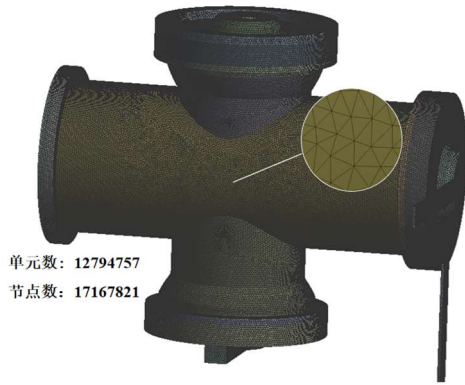
图 4 模型的网格剖分 Fig. 4 Model meshing map
